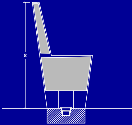
SEZIONE
